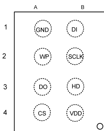
8ball WLCSP
