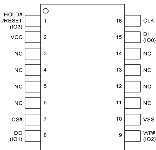
SOP16 300mil
